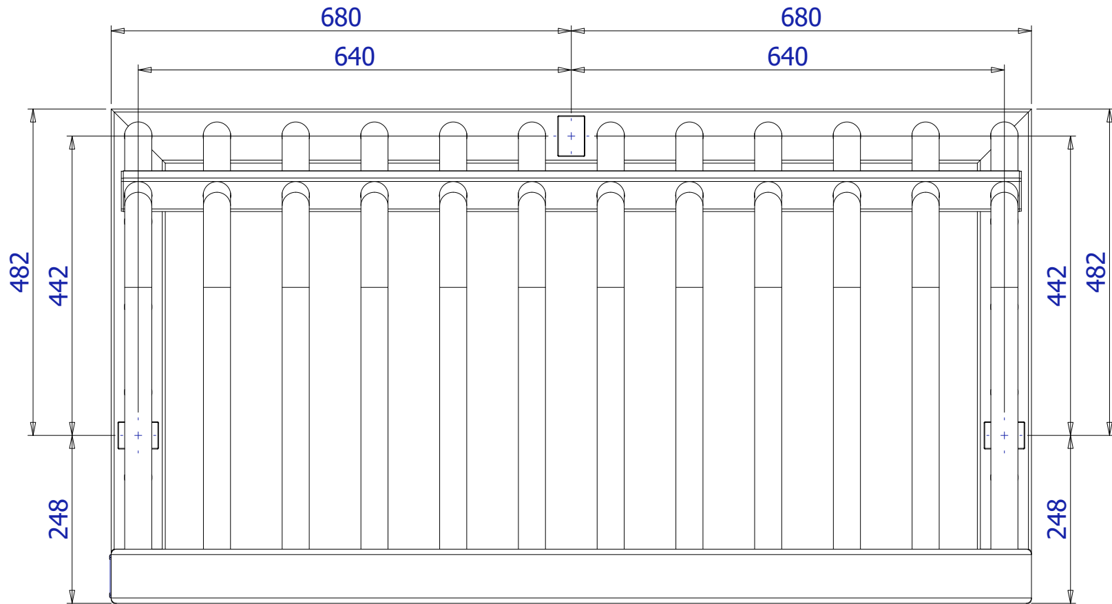
Posities van de verankeringspunten • Bovenaanzicht Anchor point positions • Top view
